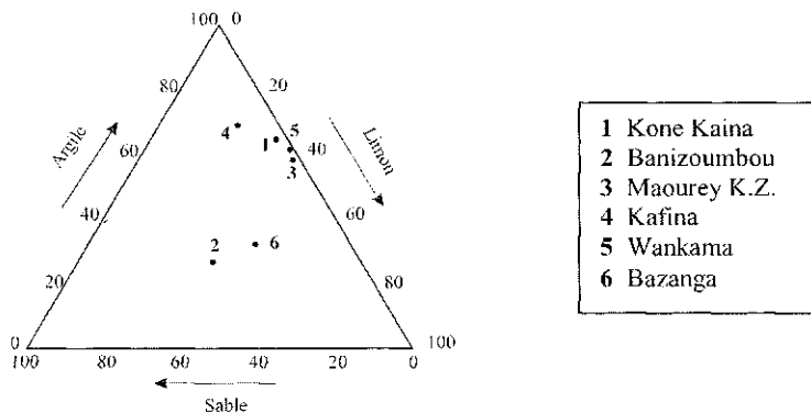
Fig. 3 Granulométrie de la zone colmatée en différentes mares de la région de Niamey.
