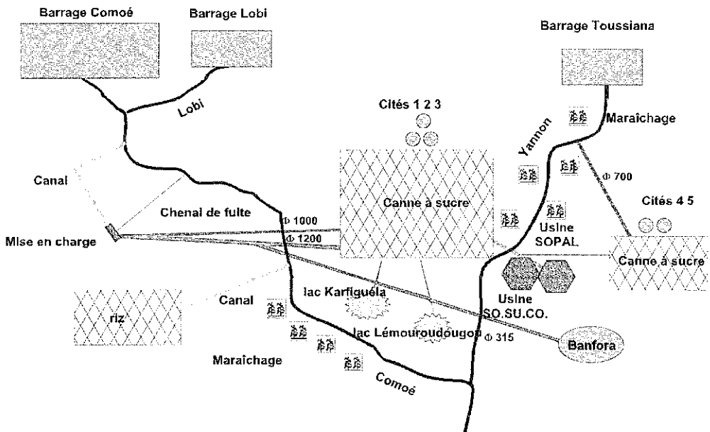
Fig. 1 Plan schématique de l'hydro-aménagement de la Comoé.
